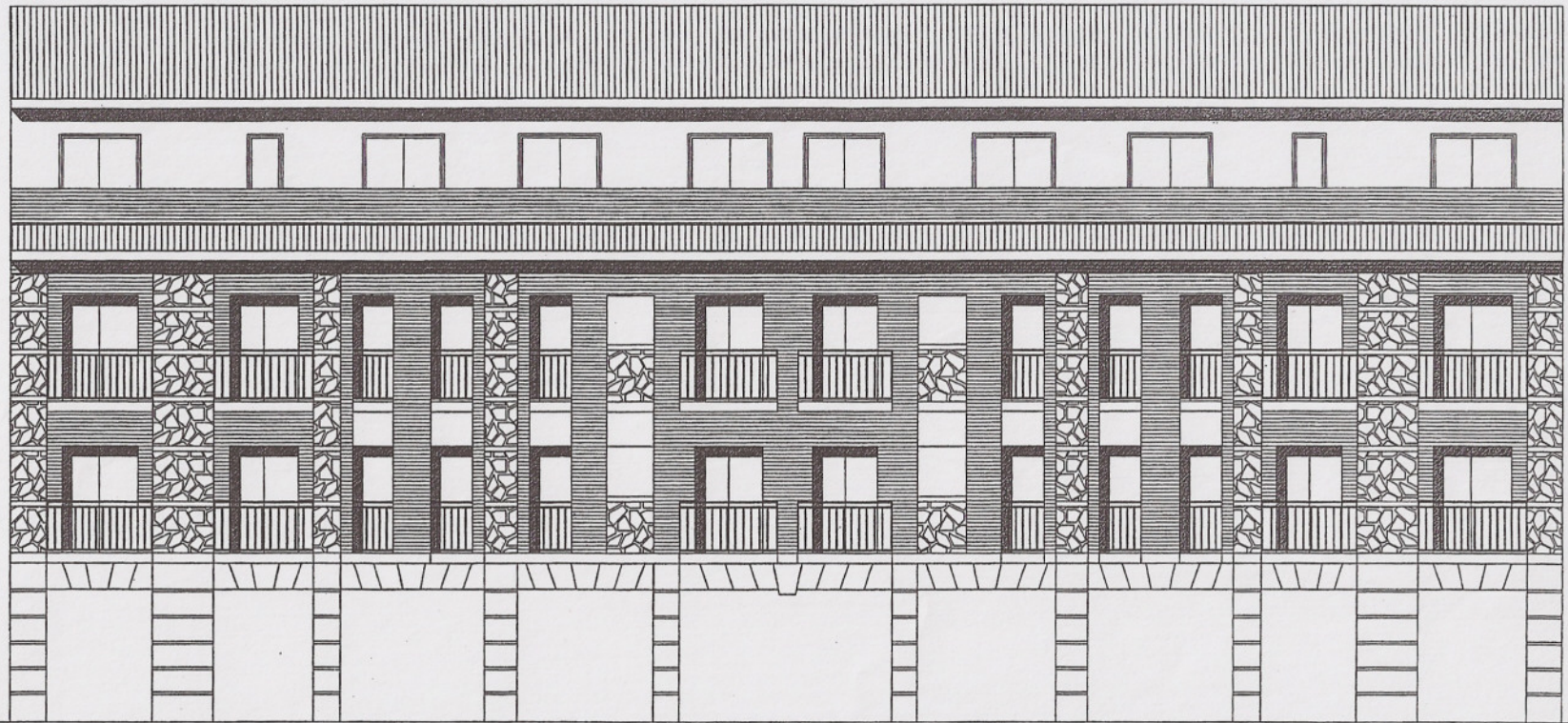
ALZADO TRAMO DE CALLE
