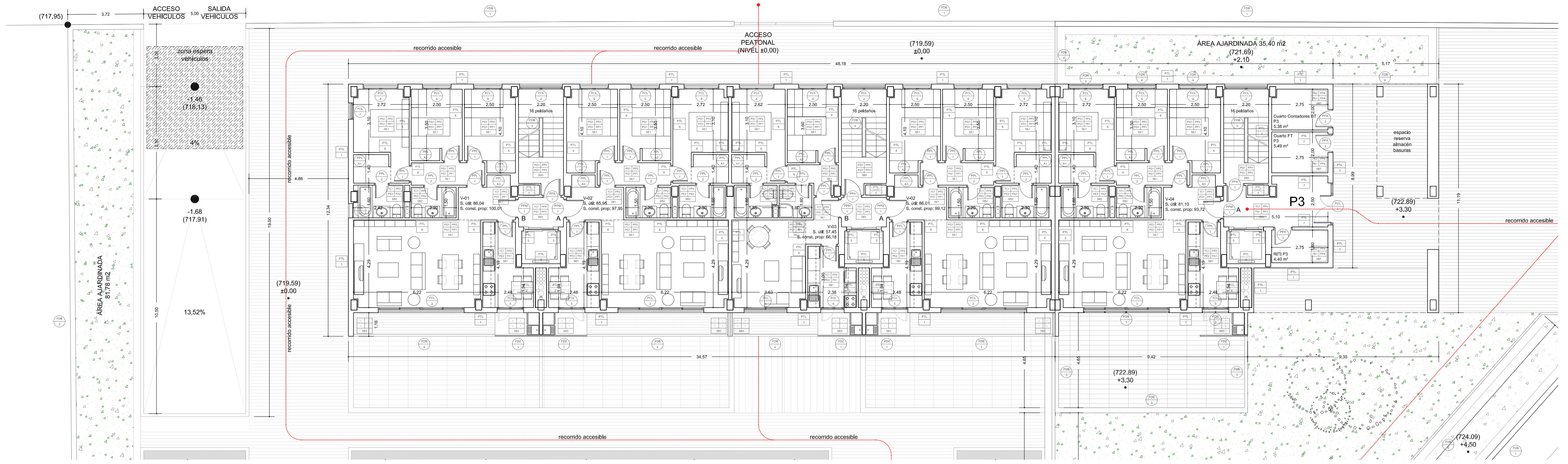
PLANTA 1ª (NIVEL +3.30) E 1/100
