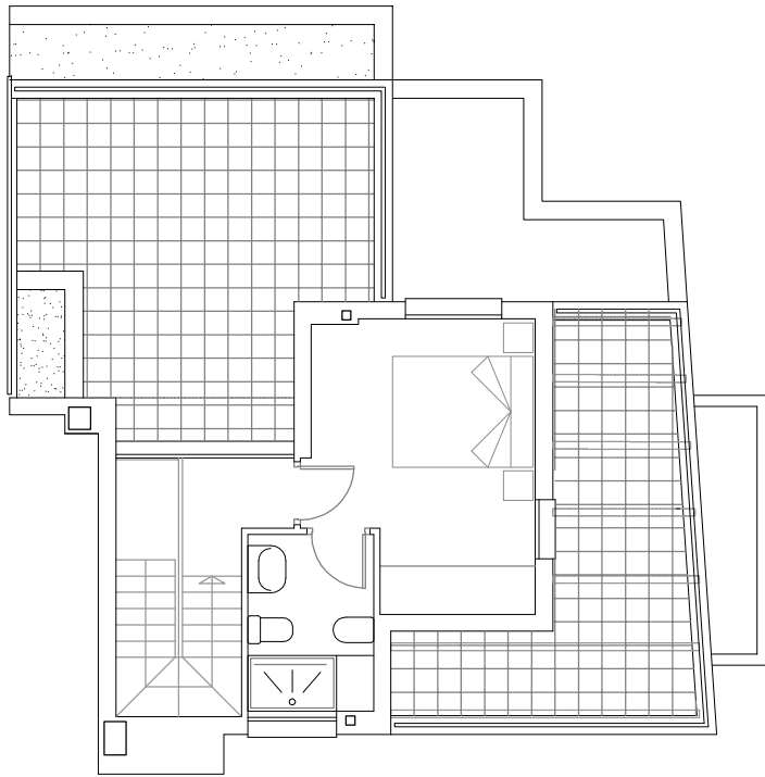
PLANTA ALTA
