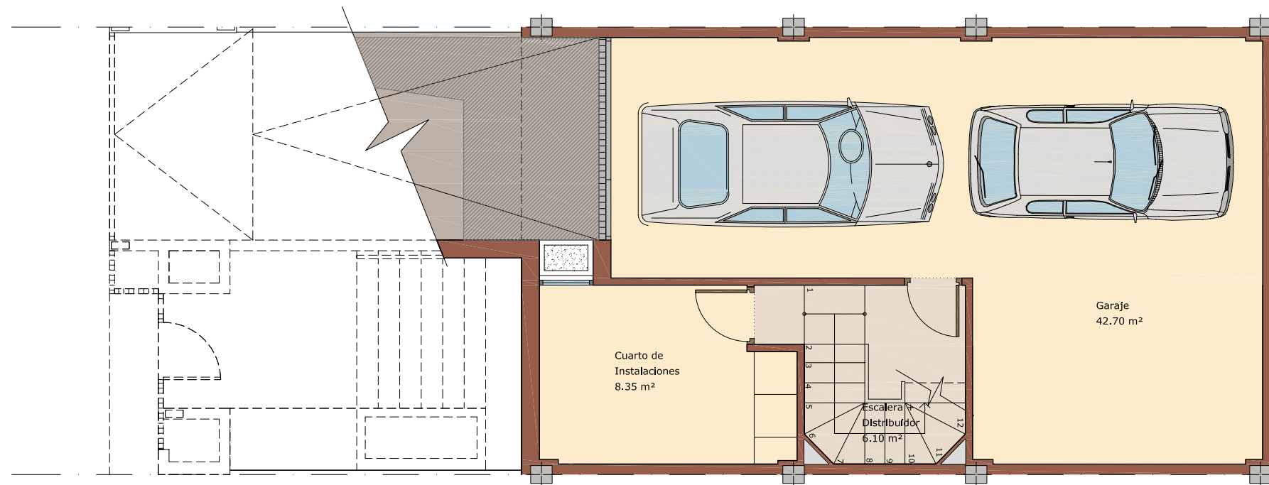
PLANTA SÓTANO ESCALA 1/75
