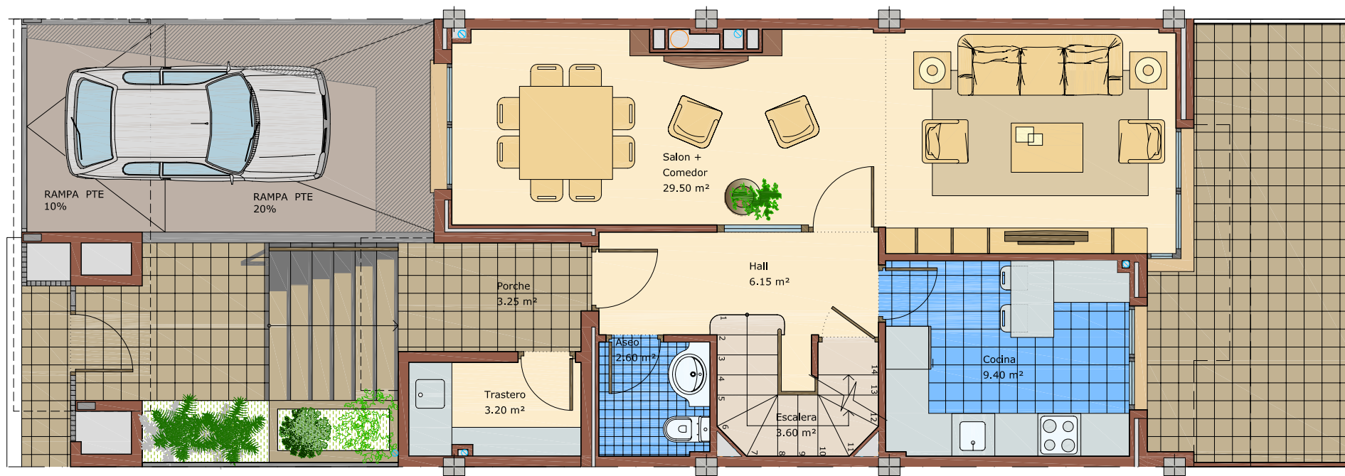
PLANTA BAJA ESCALA 1/75
