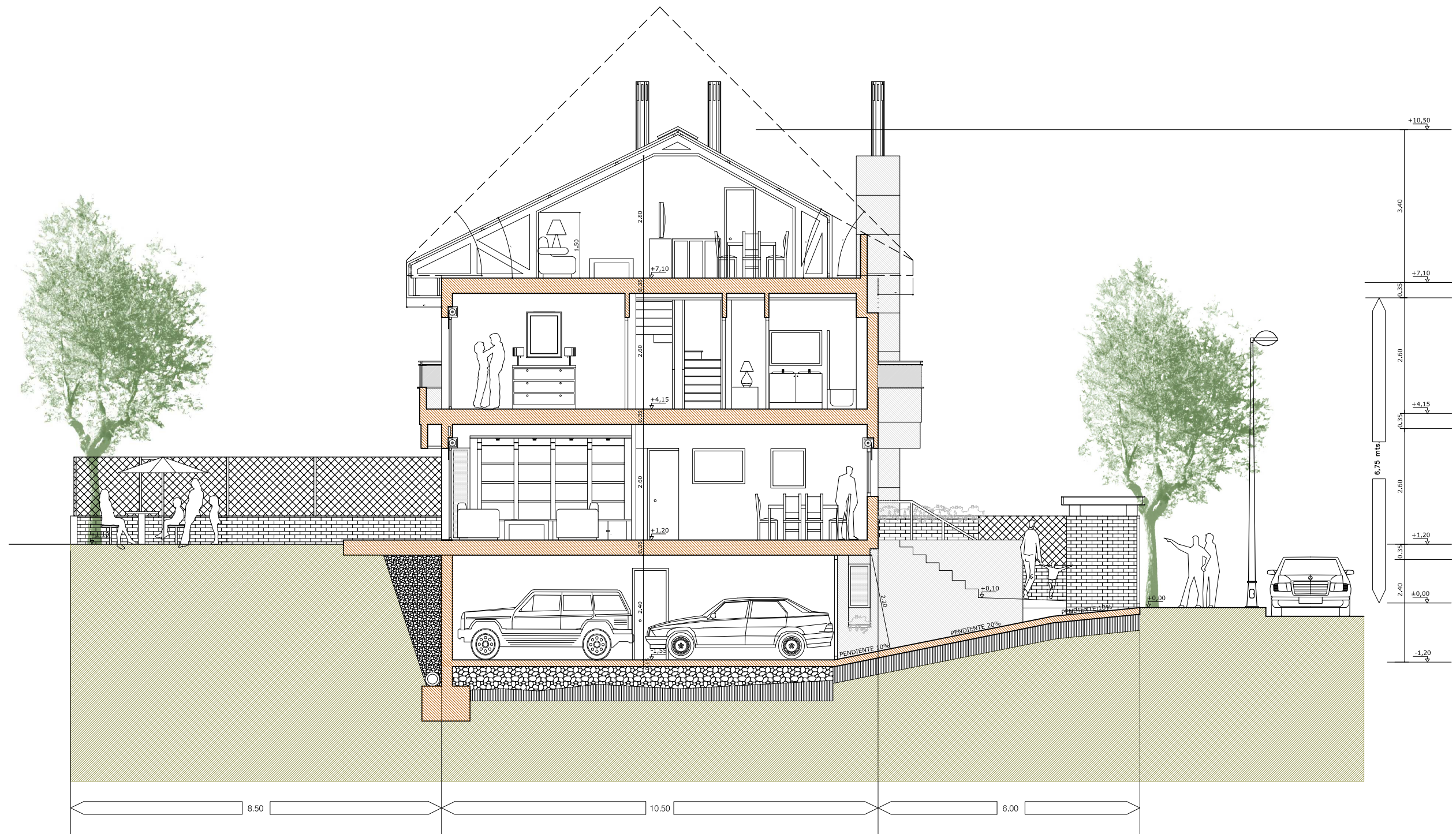
SECCION LONGUITUDINAL 1/100
