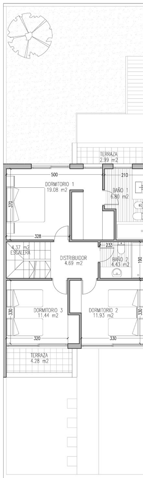
PLANTA PRIMERA 72.00 m 2
