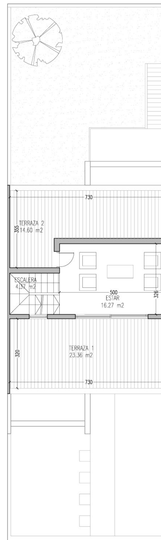
PLANTA ATICO 24.72 m 2
