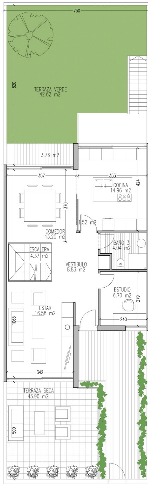
PLANTA BAJA 78.28 m 2
