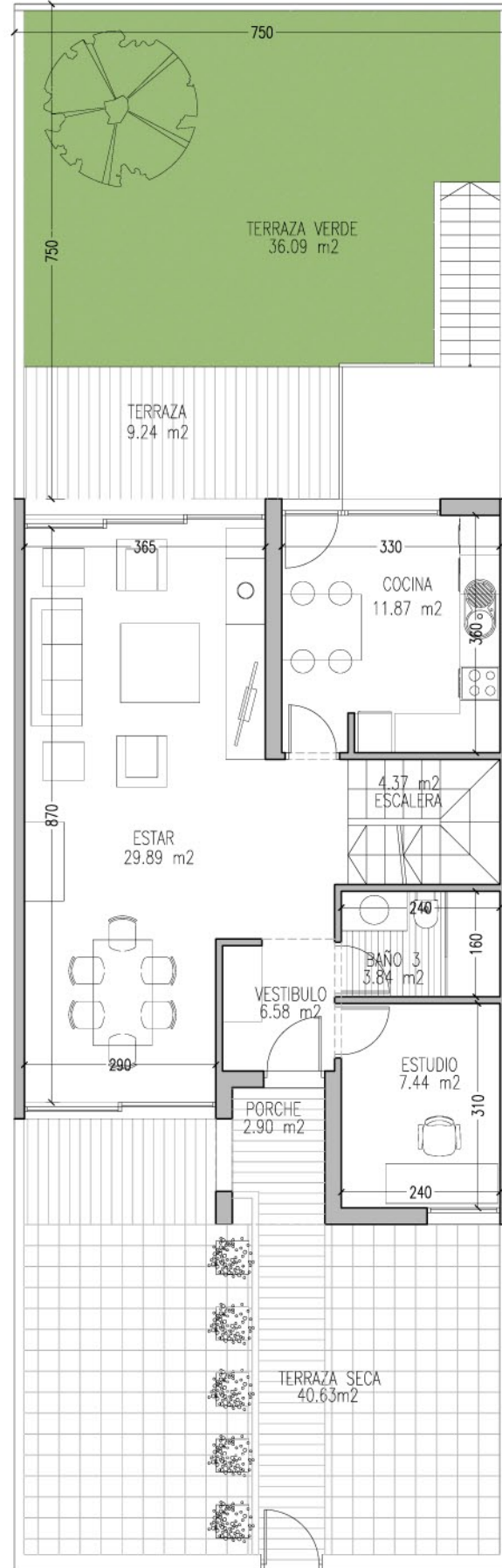
PLANTA BAJA 74.32 m 2
