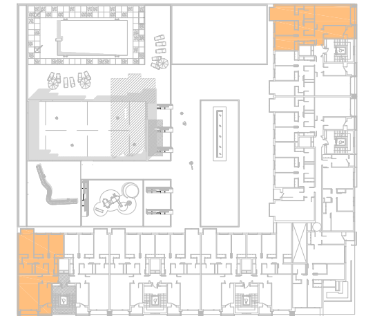
PLANTA TIPO (1º A 6º) Y 7º
