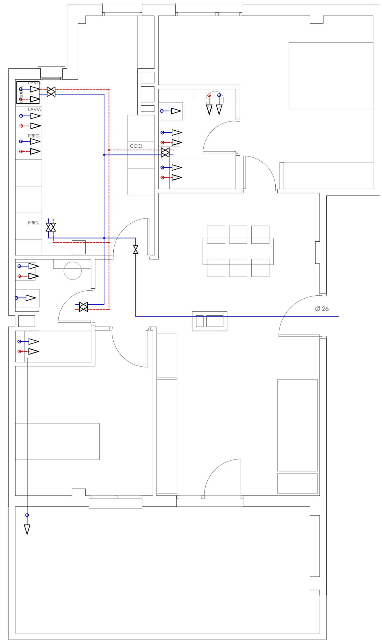
VIVIENDA TIPO 16 (6 uds.) 041A - 024B - 034A - 044B - 054A - 064B
