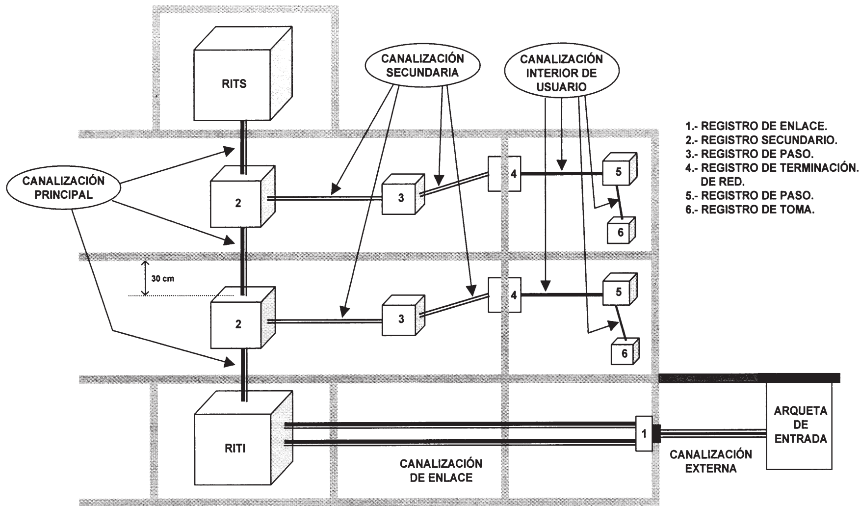
APÉNDICE 2: ESQUEMA DE CANALIZACIONES PARA INMUEBLES DE PISOS
