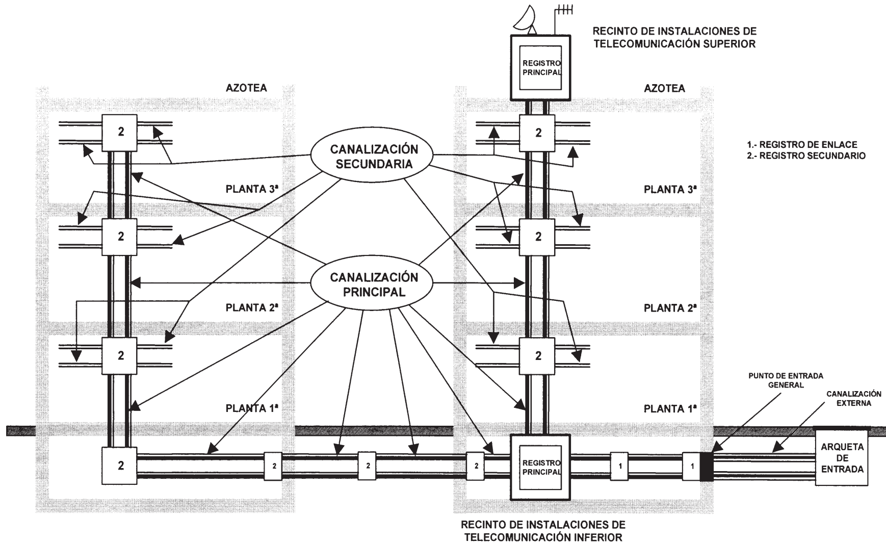
APÉNDICE 6: EJEMPLO DE ESQUEMA GENERAL DE CANALIZACIÓN CON DIFERENTES VERTICALES EN EDIFICIOS INDEPENDIENTES
