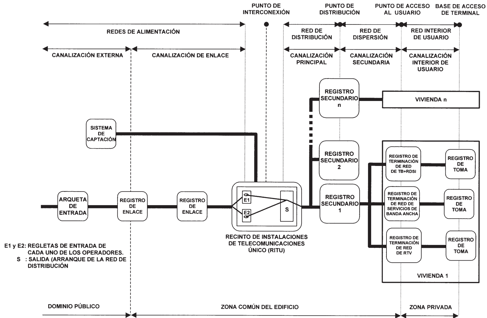
APÉNDICE 8: ESQUEMA GENERAL DE UNA ICT PARA AGRUPACIONES DE VIVIENDAS UNIFAMILIARES
