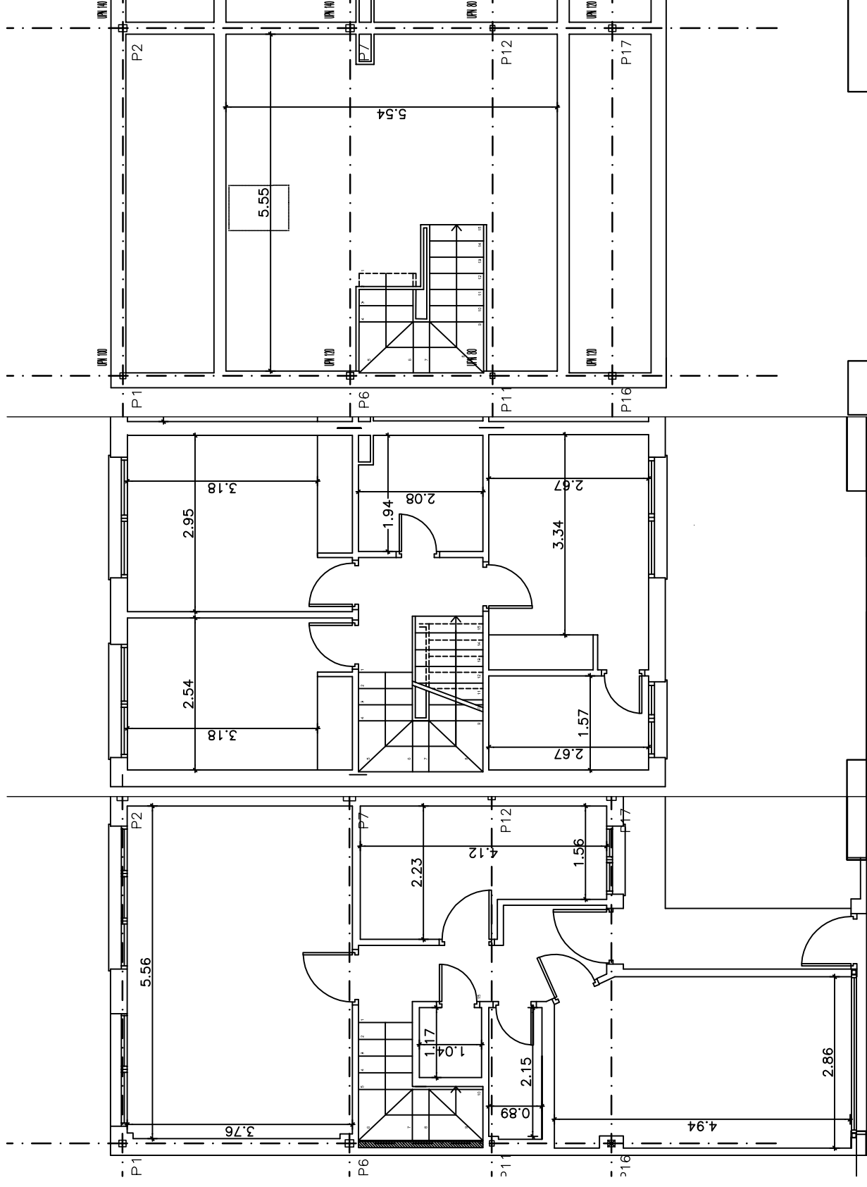
PLANTA BAJA
