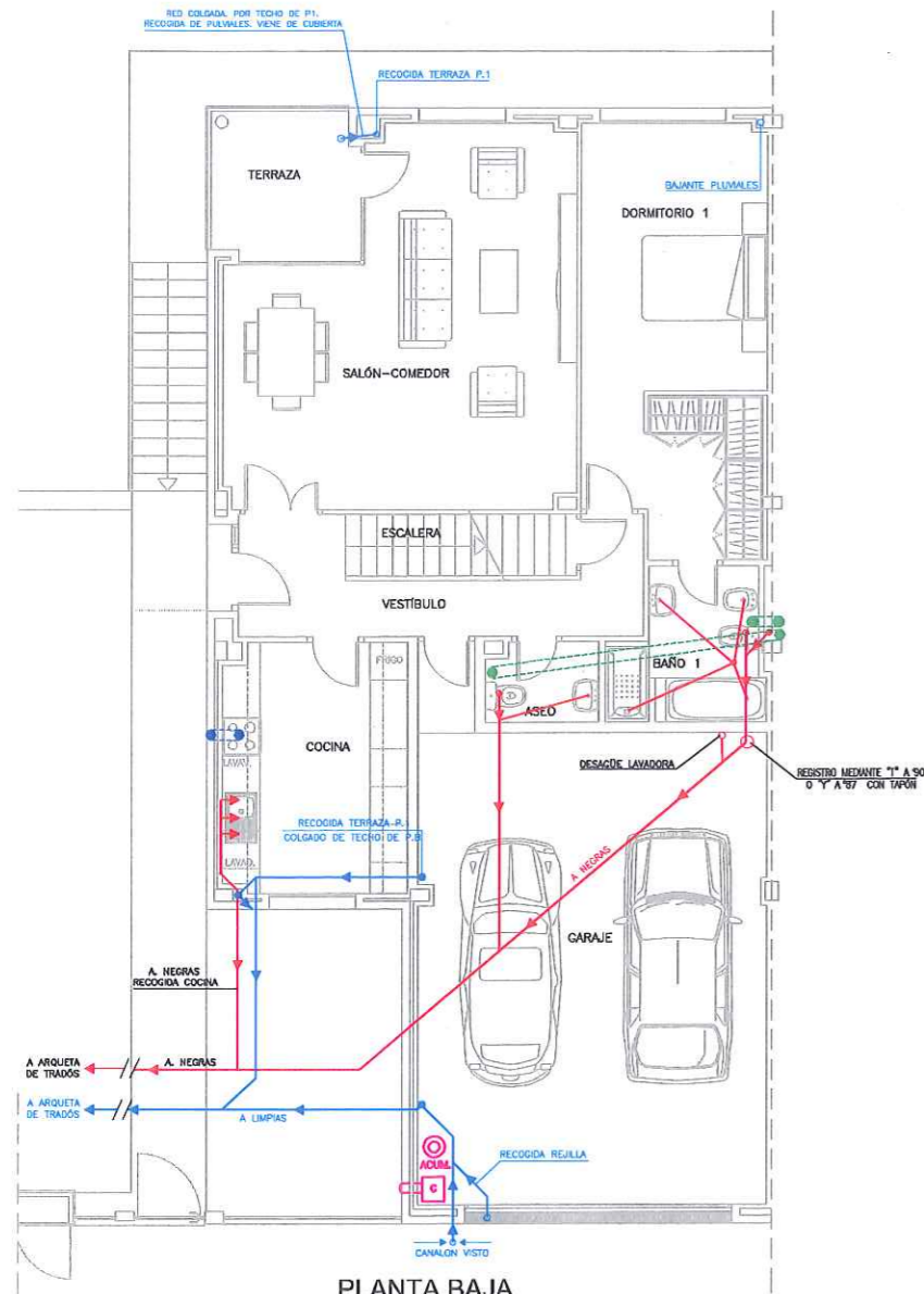
PLANTA BAJA SALÓN-COMEDOR + 1 DORMITORIO
