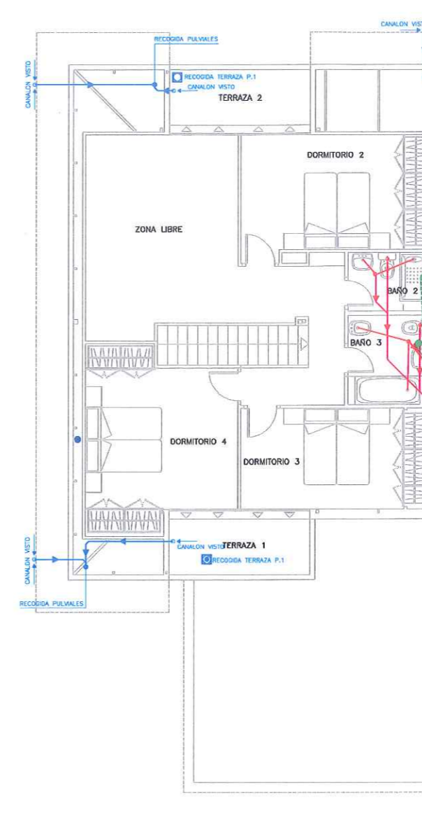
PLANTA PRIMERA 3 DORMITORIOS + ZONA LIBRE (salón-comedor + 1 dormitorio en planta baja)
