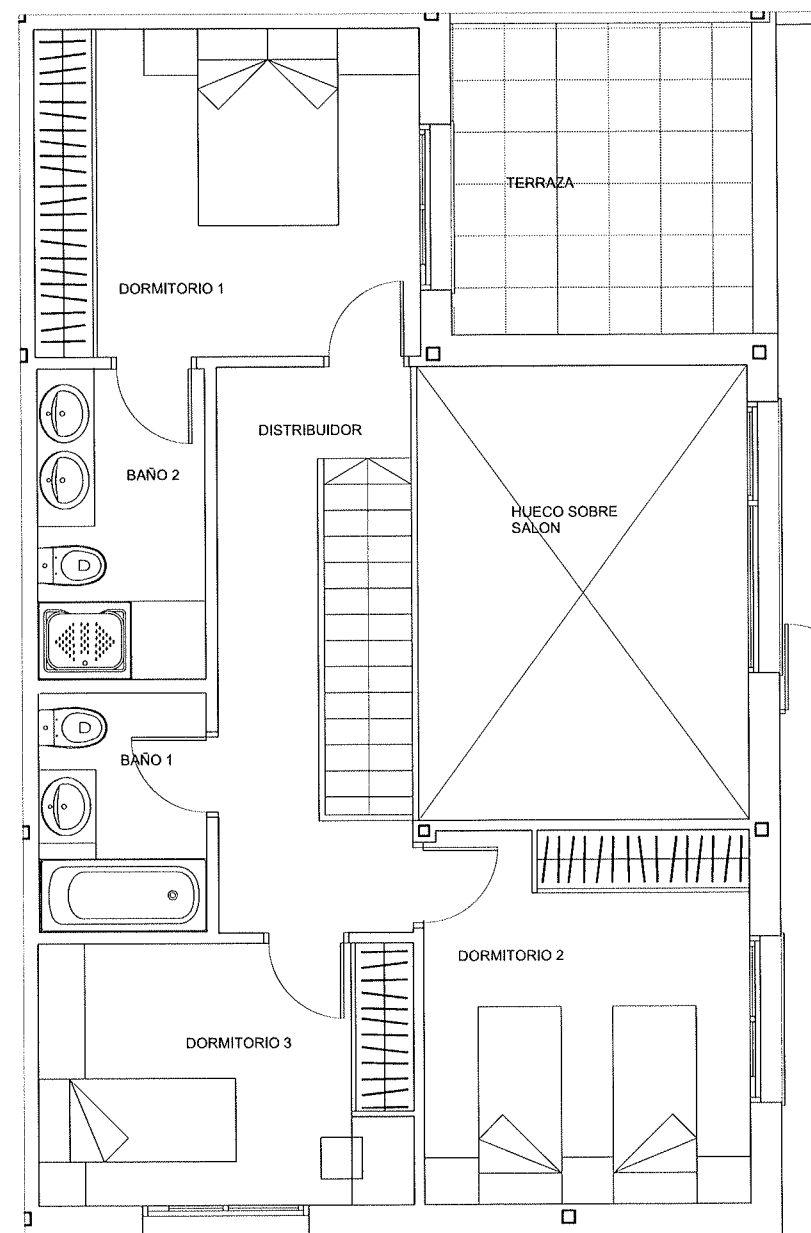
PLANTA PISO
