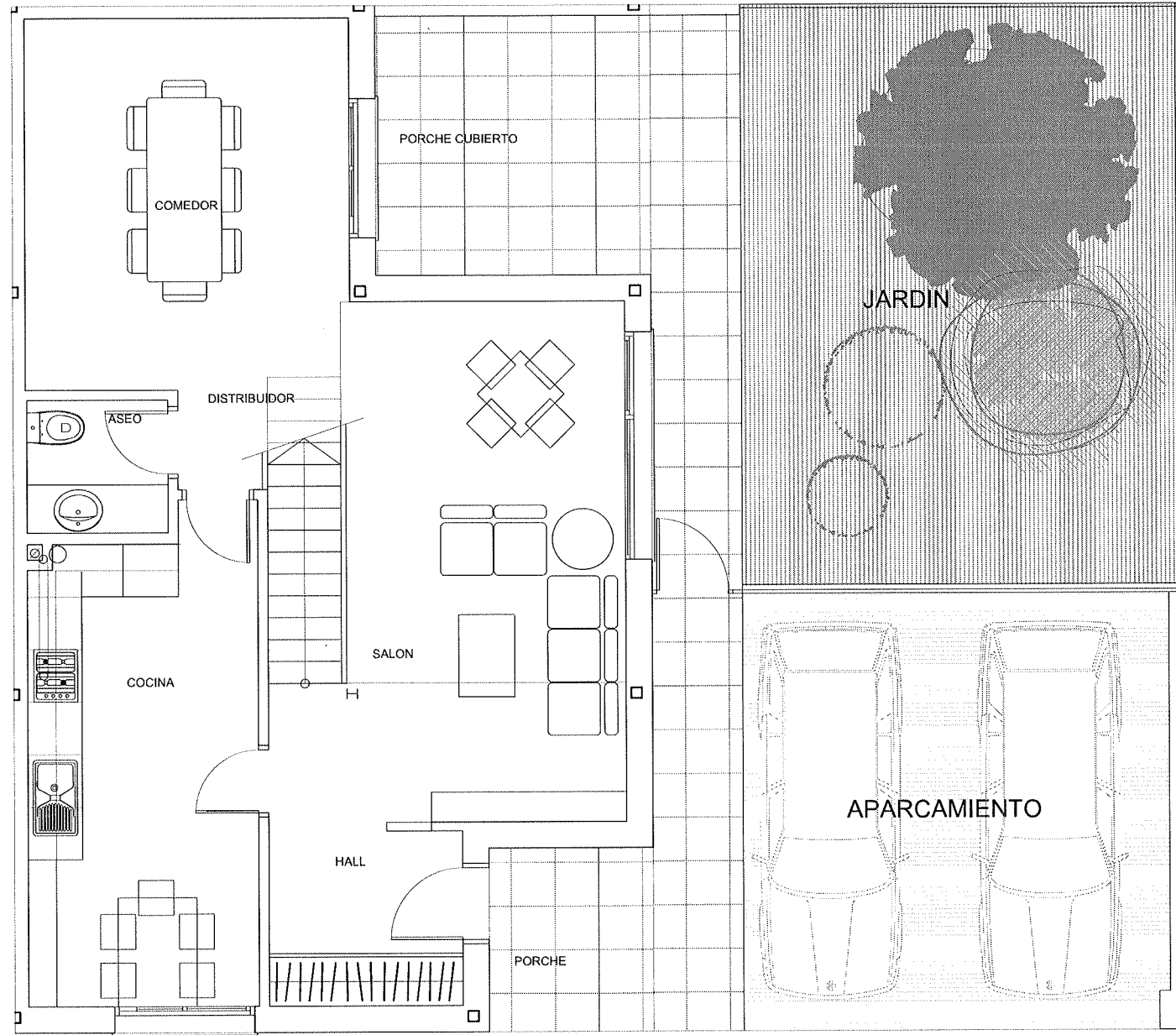
PLANTA BAJA
