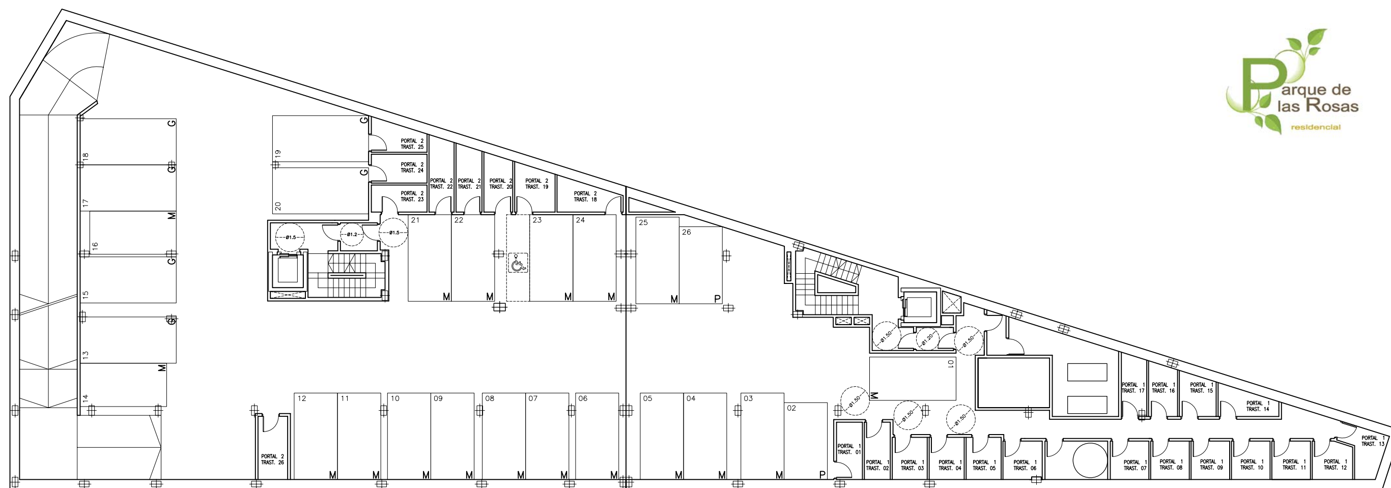
PLANTA SÓTANO 1
