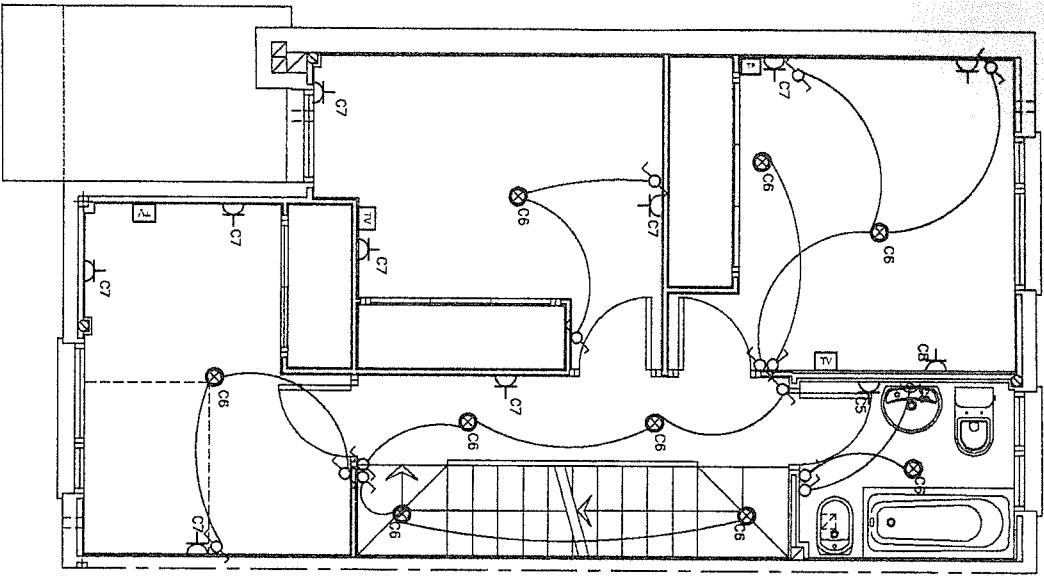
PLANTA PRIMERA
