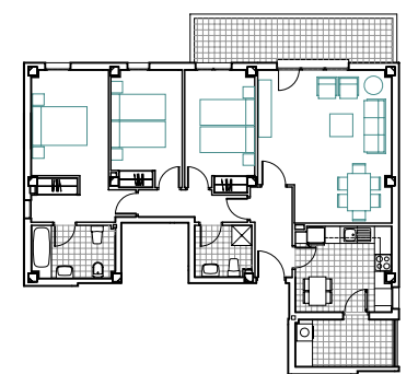
VT09 Parcela B 2 UDS. UTIL 93,56m 2
