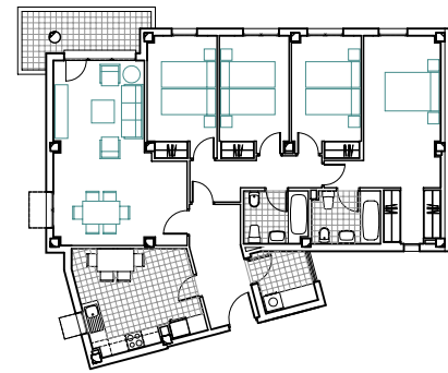
VT08 Parcela A 2 UDS. UTIL 115,97m 2
