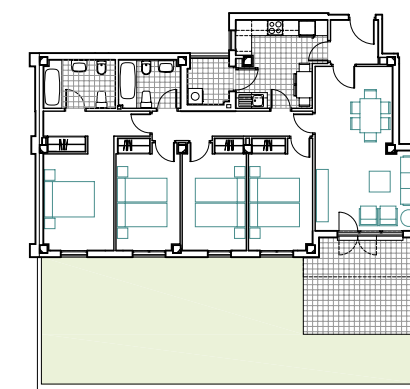
VT09 Parcela A 2 UDS. UTIL 107,49m 2
