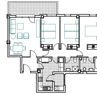
VT06 Parcela B 4 UDS. UTIL 90,41m 2
