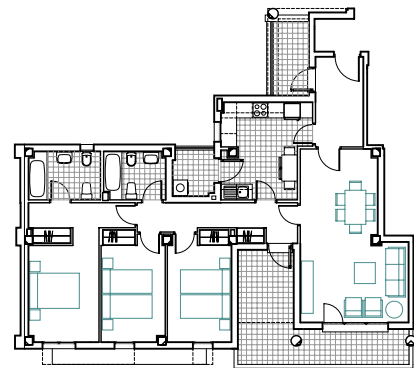
VT10 Parcela B 2 UDS. UTIL 103,14m 2
