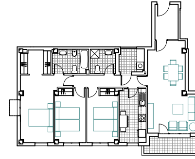
VT03 Parcela B 4 UDS. UTIL 98,41m 2
