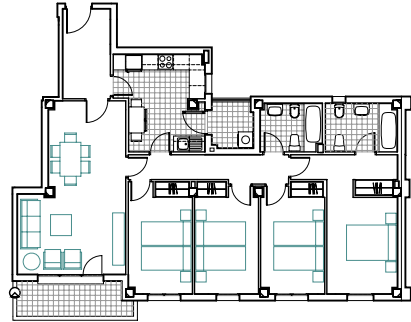
VT02 40 UDS. UTIL 107,25m 2
