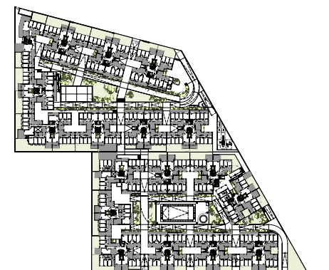
Planta Baja Parcelas 1A y 1B
