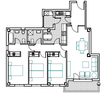
VT04 6 UDS. UTIL 92,04m 2
