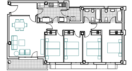
VT07 Parcela A 2 UDS. UTIL 107,74m 2
