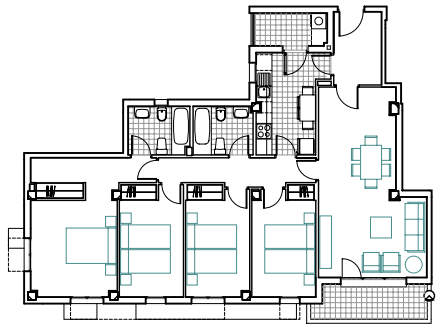
VT05 Parcela A 2 UDS. UTIL 108,39m 2
