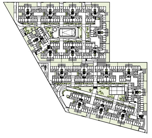
Planta Baja Parcelas 1A y 1B
