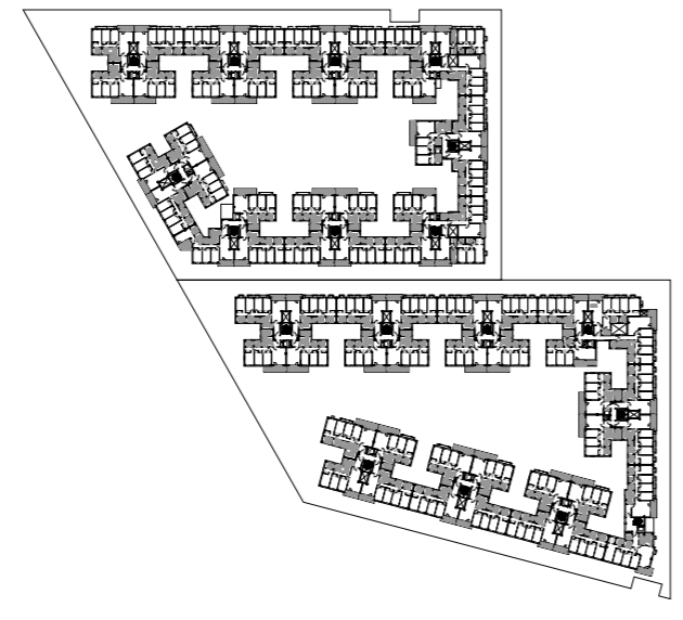
Planta Primera Parcelas 1A y 1B
