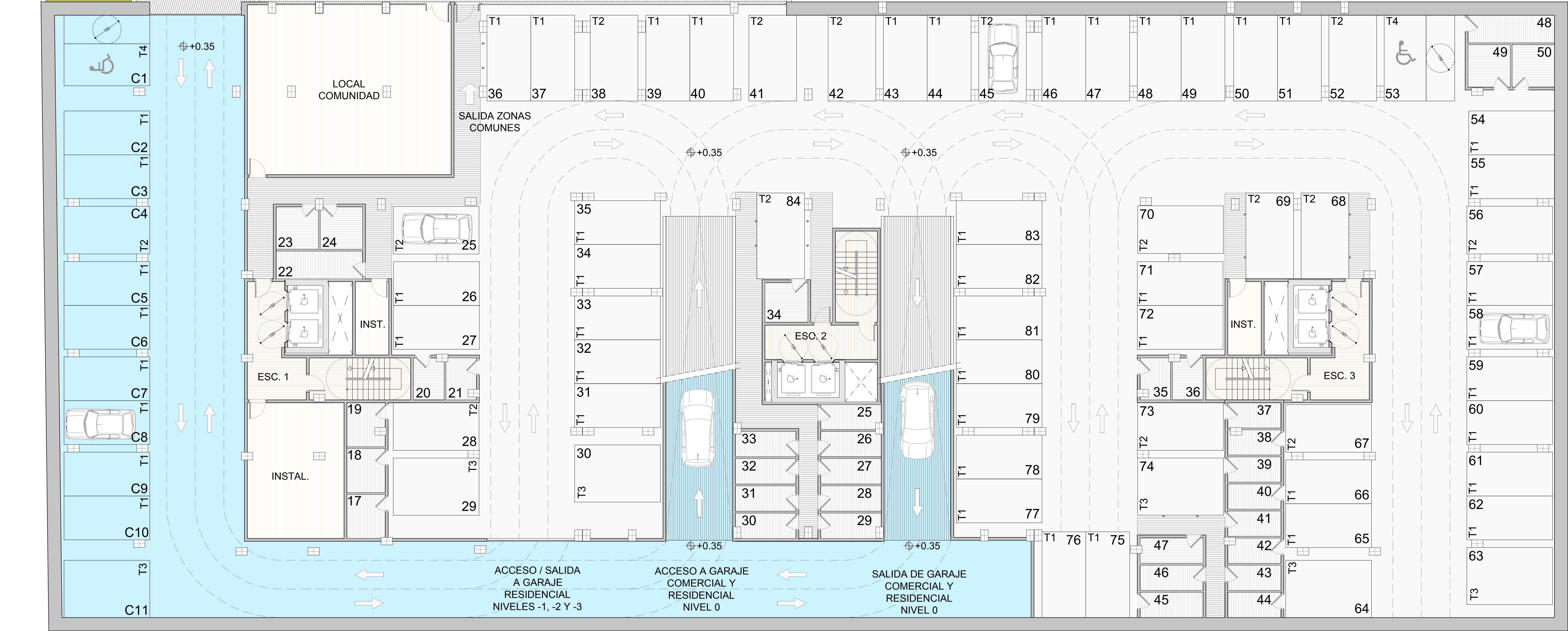
PLANTA SÓTANO -1
