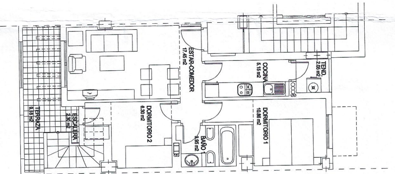
PLANTA SEGUNDA
