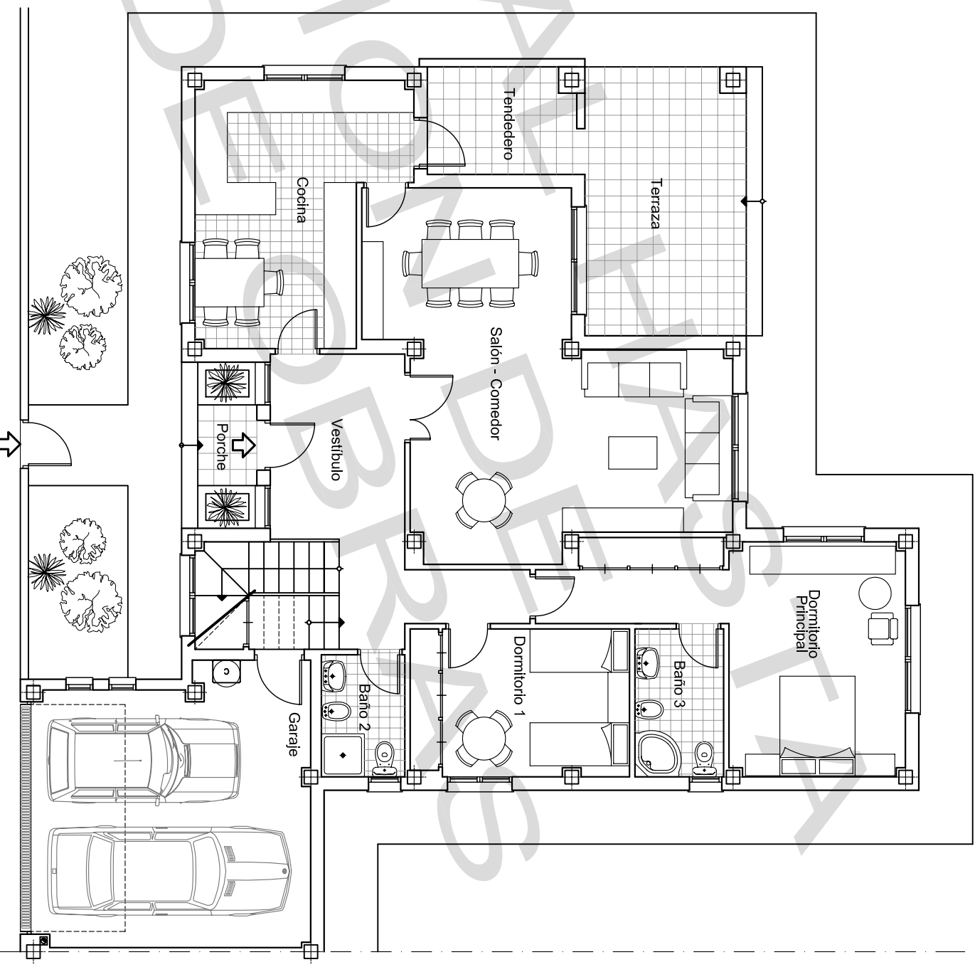
PLANTA BAJA
