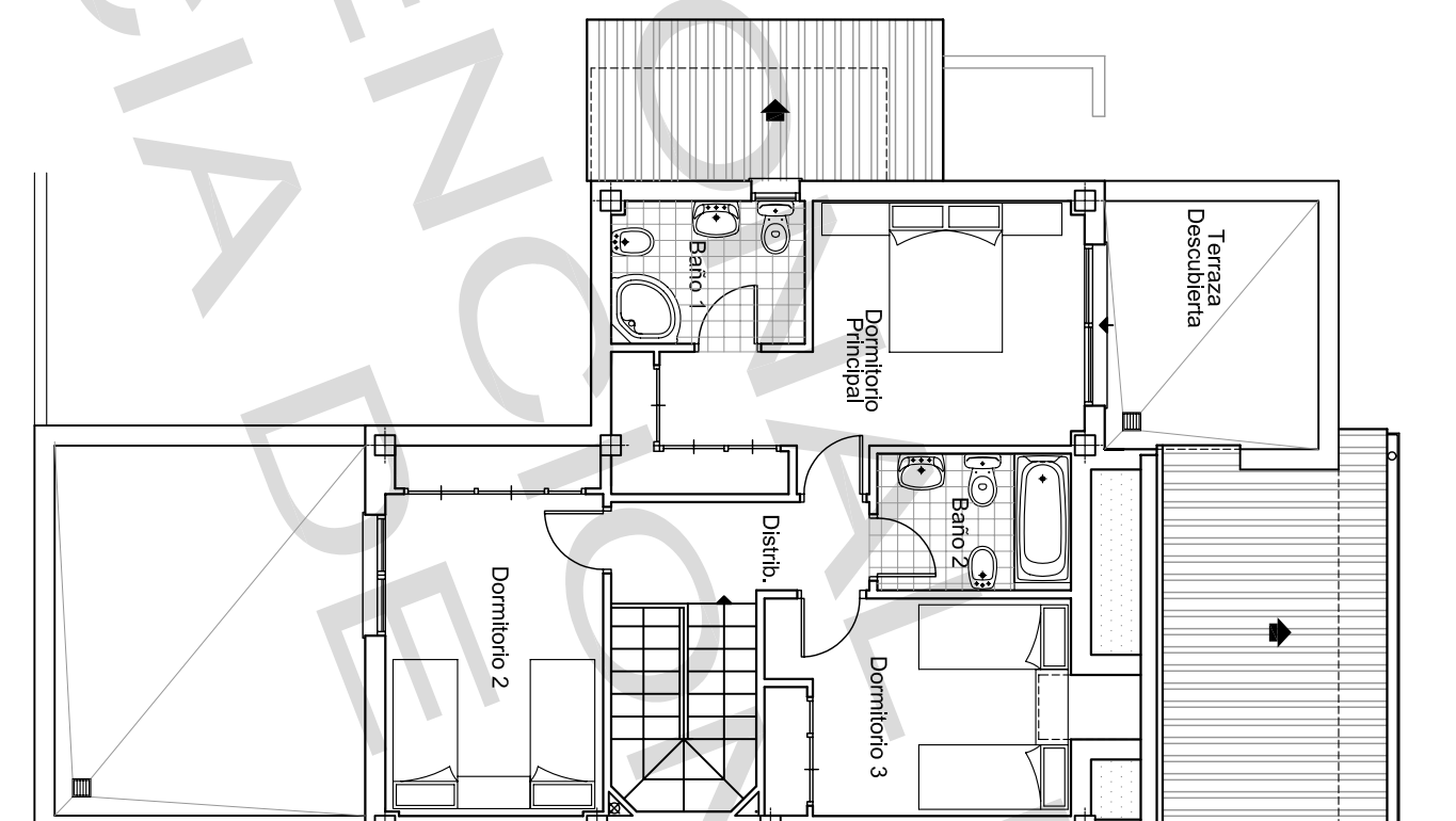
PLANTA PRIMERA
