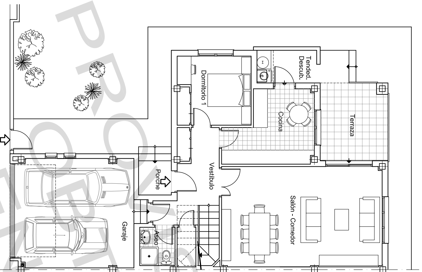
PLANTA BAJA
