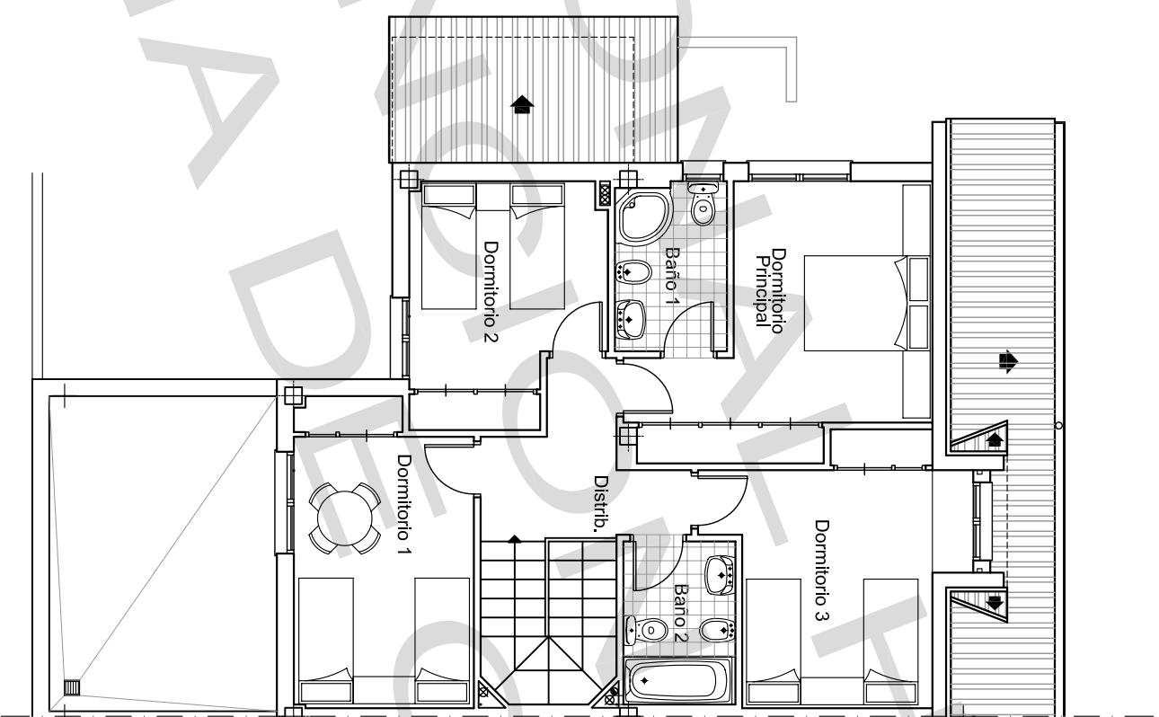
PLANTA PRIMERA
