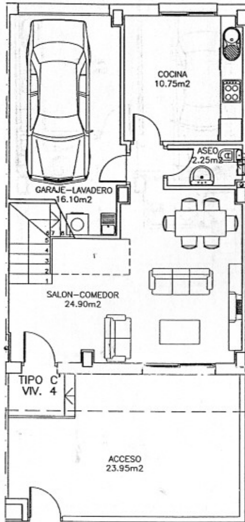
PLANTA BAJA
