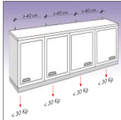
Fig. 2: reparto de la carga.
