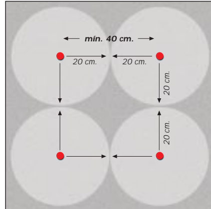
Fig. 1: separación mínima entre anclajes.
