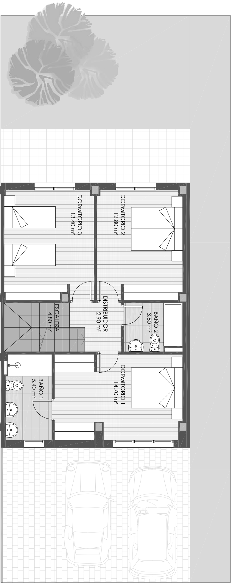
Primera planta
