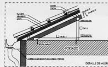
DETALLE DE ALERO
