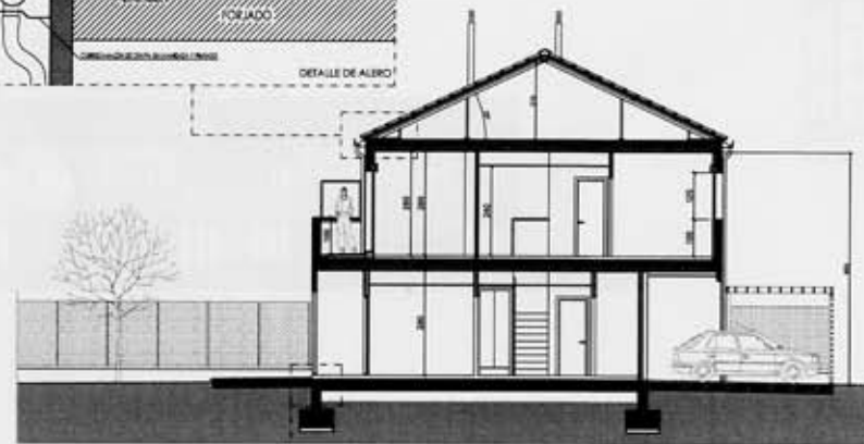
SECCION
