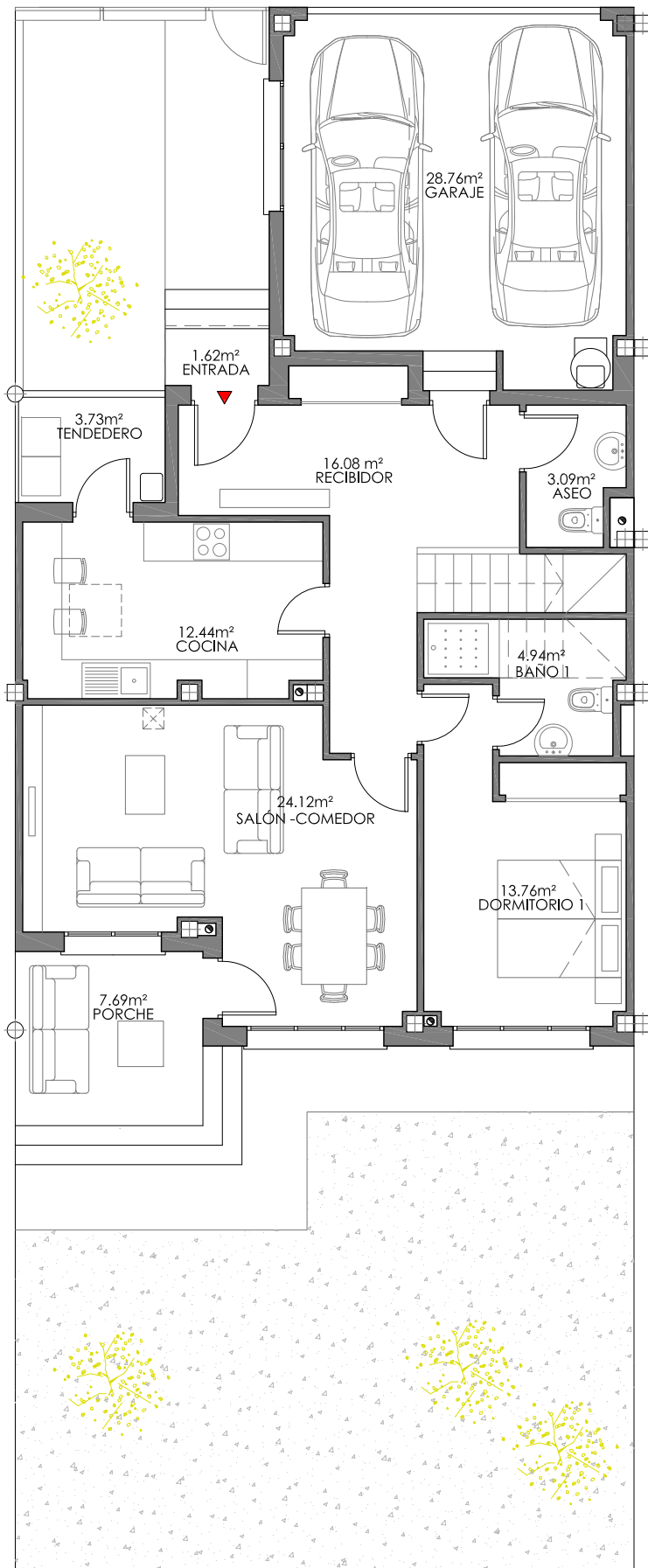
PLANTA BAJA
