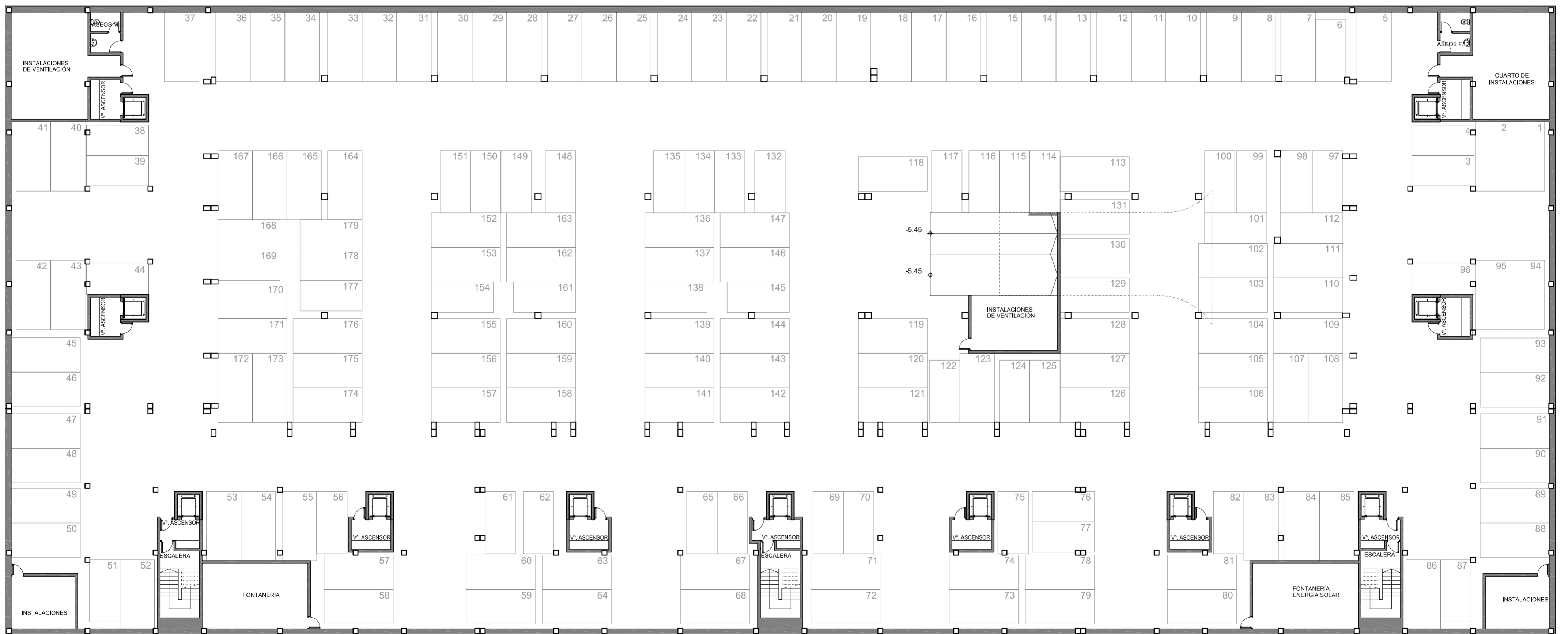
SOTANO -2
